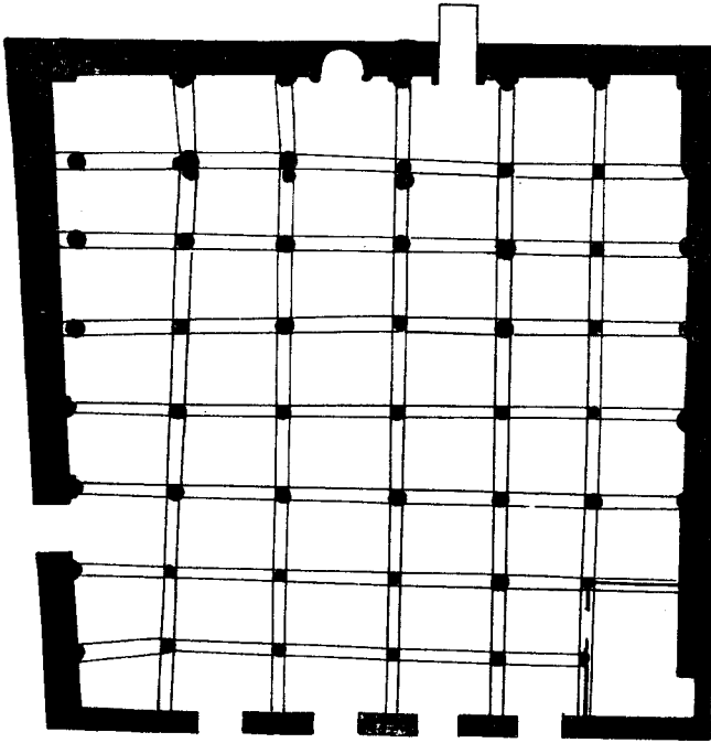
( ش38 ) مخطط غرفة الصلاة للجامع الكبير في قسطنطينة
