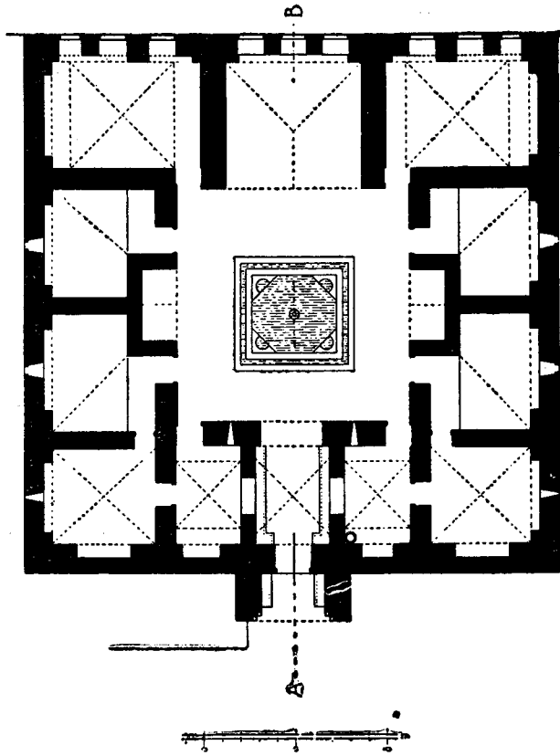
شكل ١٣ - تخطيط أساسات البجارسن القيسري عن كارل ولزنجير و كارل وتزنجير
